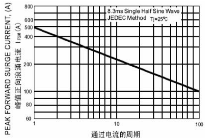
FIG. 4 – 正向特性曲线(典型)
