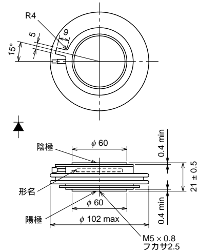
外形図
