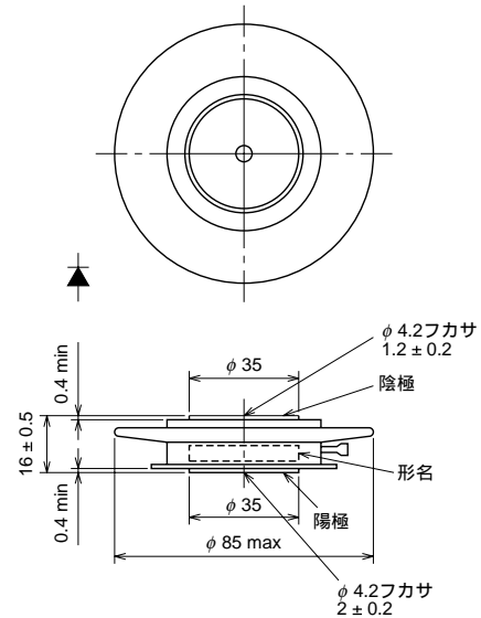
外形図
