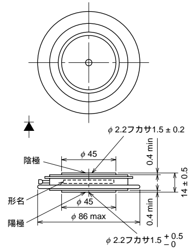
外形図
