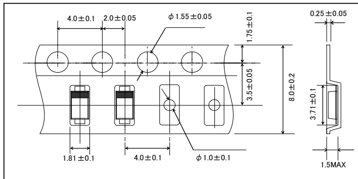
●テーピング仕様 (Unit : mm)
