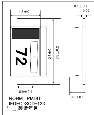
●外形寸法図 (Unit : mm)
