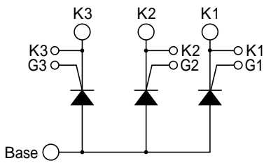
回路図 CIRCUIT
