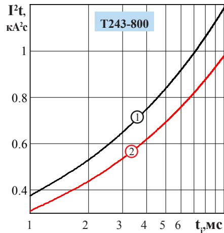
Рисунок 5 - Зависимость защитного показателя I^2t от длительности импульса тока t_p при температуре T_j = 25\text{ }^\circ\text{C} (1) и максимальной температуре перехода T_{jm} (2)
