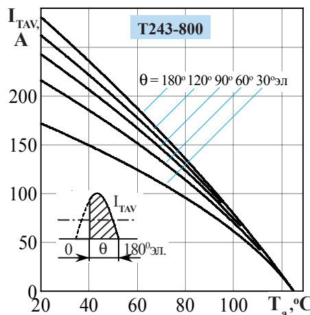
Рисунок 8 - Зависимость допустимого среднего тока в открытом состоянии I_{TAV} от температуры окружающей среды T_a при естественном охлаждении на охлаждающем устройстве ОР243-150 при различных углах проводимости для токов синусоидальной формы частотой 50 \text{ Гц}
