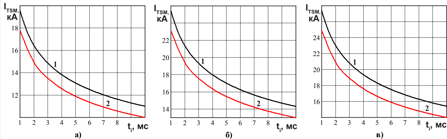
Рисунок 4 - Зависимость допустимой амплитуды ударного тока в открытом состоянии I_{TSM} от длительности импульса тока t_i при исходной температуре структуры T_j = 25 °C (1) и максимально допустимой температуре перехода T_{jm} (2) для модулей:
