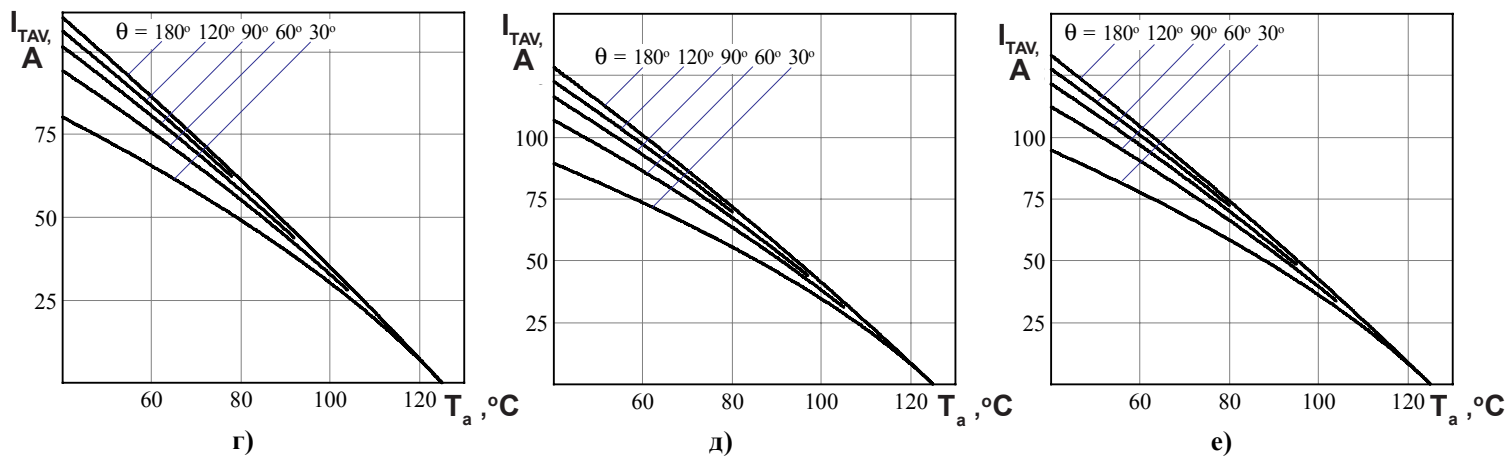
Рисунок 8 - Зависимость допустимого среднего тока в открытом состоянии I_{TAV} синусоидальной формы частотой 50 Гц при различных углах проводимости от температуры окружающей среды T_a при естественном охлаждении для модулей:
