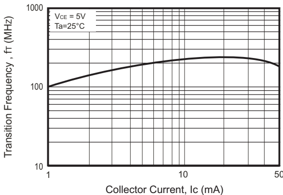
Fig.7- f_r - I_c
