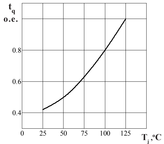
Рисунок 11 - Зависимость времени выключения t_q от температуры структуры T_j при I_T = I_{TAVM} ; U_R = 100 В; di_T/dt = 5 А/мкс; dU_D/dt = 50 В/мкс
