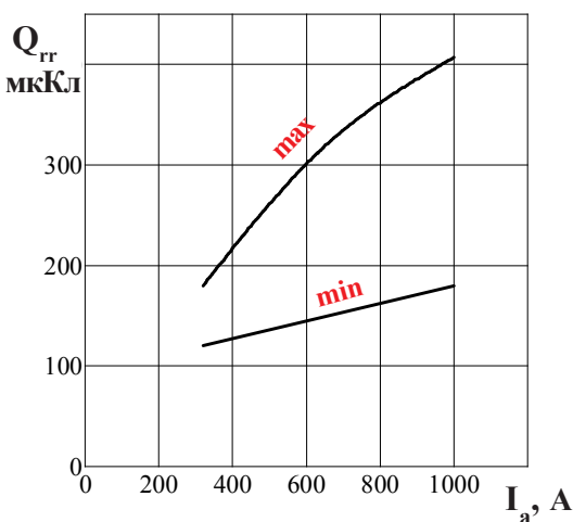
Рисунок 14 - Зависимость заряда восстановления Q_{rr} от анодного тока I_a при T_{jm} = 125 °С; I_T = I_{T(AV)} ; di_T/dt = 50 А/мкс
