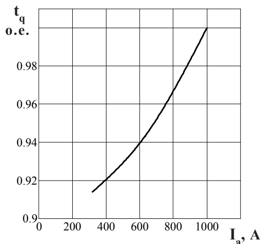
Рисунок 15 - Зависимость времени выключения t_q от анодного тока I_a при T_{jm} = 125 °С; I_T = I_{T(AV)} ; di_T/dt = 5 А/мкс; dU_D/dt = 50 В/мкс
