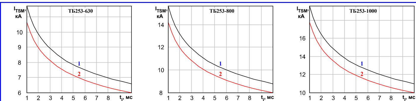
Рисунок 4: Зависимость допустимой амплитуды ударного тока I_{TSM} от длительности импульса тока t_i при исходной температуре структуры T_j=25^\circ\text{C} (1) и максимально допустимой температуре перехода T_{jm} (2).
