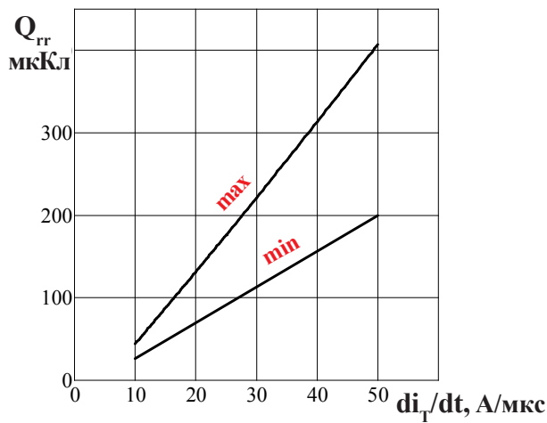
Рисунок 12 - Зависимость заряда восстановления Q_{rr} от скорости спада тока di_T/dt в открытом состоянии при температуре перехода T_{jm} = 125 °С; U_R = 100 В; I_T = I_{T(AV)}
