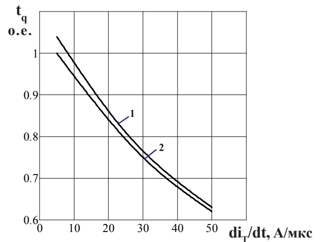
Рисунок 13 - Зависимость времени выключения t_q от скорости спада тока в открытом состоянии di_T/dt при T_{jm} = 125 °С; I_T = I_{T(AV)} ; U_R = 100 В; 1 - при dU_D/dt = 100 В/мкс; 2 - при dU_D/dt = 50 В/мкс
