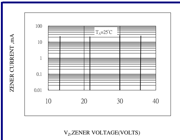
Fig.3B-V Z =12 THRU 36 VOLTS
