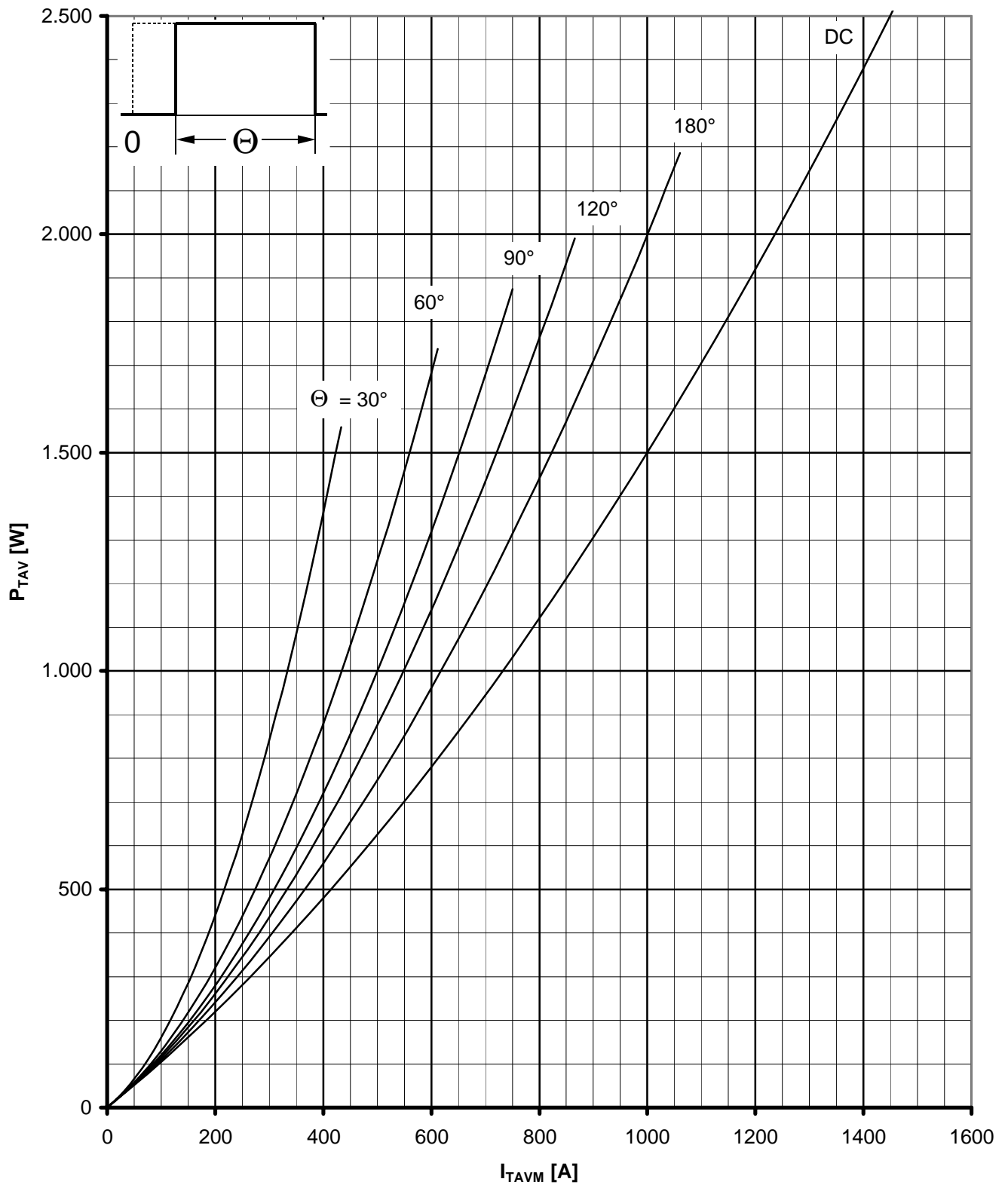
Durchlaßverlustleistung / On-state power loss P_{TAV} = f(I_{TAVM}) Parameter: Stromflußwinkel \Theta / current conduction angle \Theta
