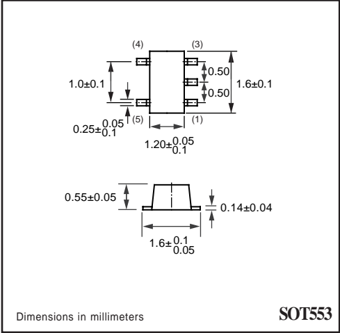
SOT553
