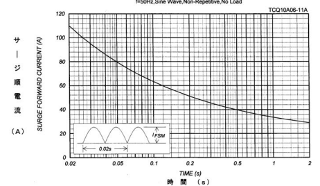
サージ順電流定格 SURGE CURRENT RATINGS
