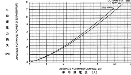
平均順電力損失特性 AVERAGE FORWARD POWER DISSIPATION
