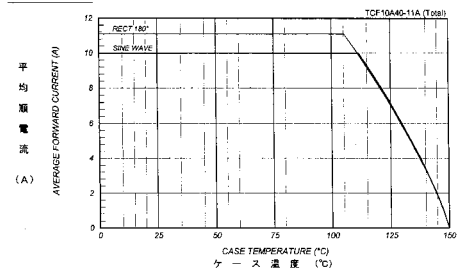
平均順電流 - ケース温度定格 AVERAGE FORWARD CURRENT VS. CASE TEMPERATURE
