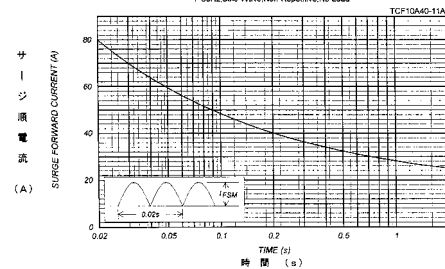
サージ順電流定格 SURGE CURRENT RATINGS
