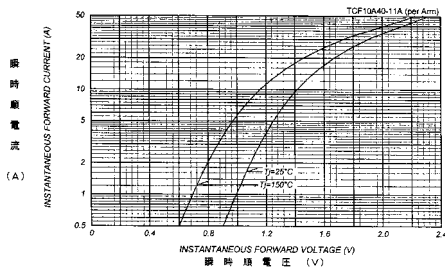
順電圧特性 FORWARD CURRENT VS. VOLTAGE
