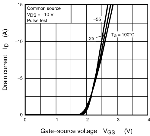
Fig. 8.1.3 I_D - V_{GS}
