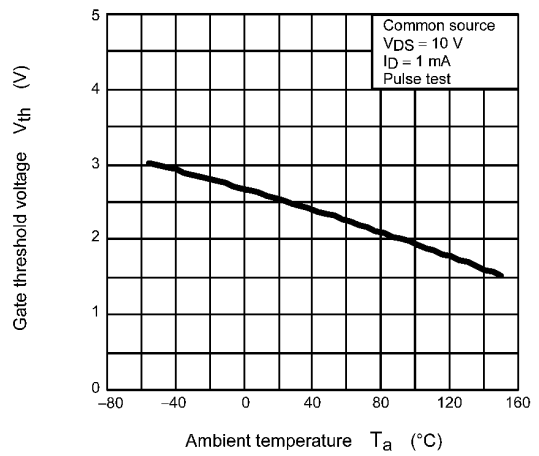
Fig. 8.10 V_{th} - T_a
