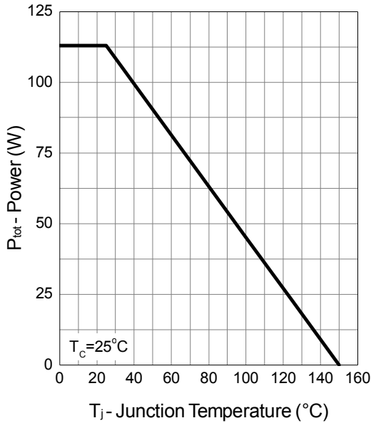
Power Dissipation : TO-220/TO-251
