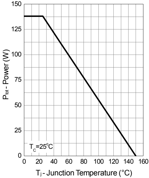
Power Dissipation : TO-220/TO-247
