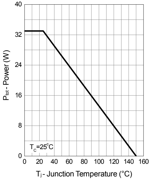
Power Dissipation : TO-220/TO-252
