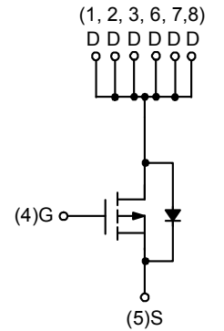
P-Channel MOSFET
