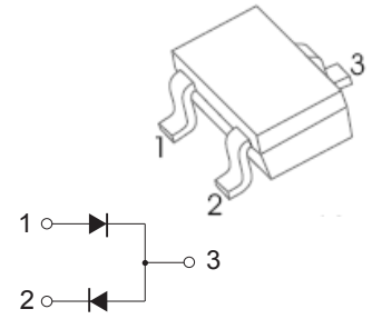
SOT-323
