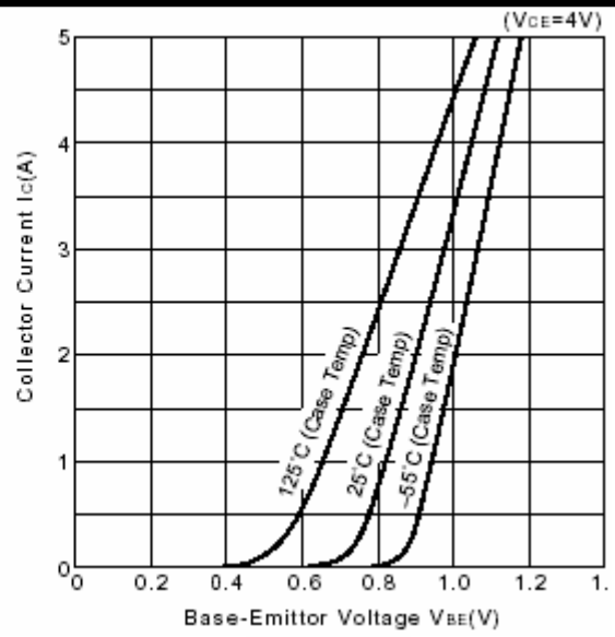
Fig.4 I_C - V_{BE}
