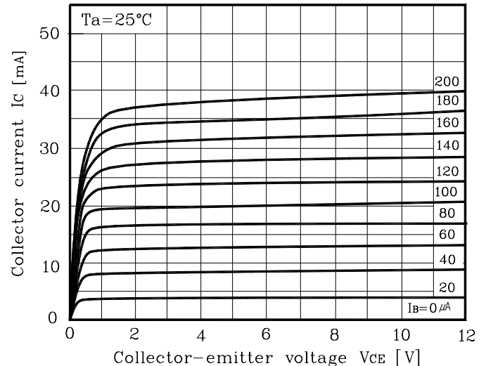
Fig. 2 I_C - V_{CE}
