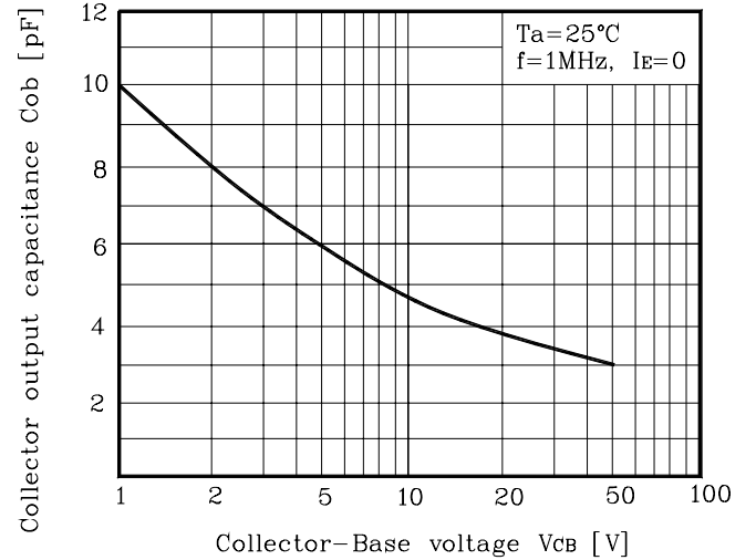
Fig. 4 C_{ob} - V_{CB}
