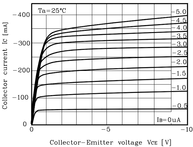
Fig. 3 I_C - V_{CE}
