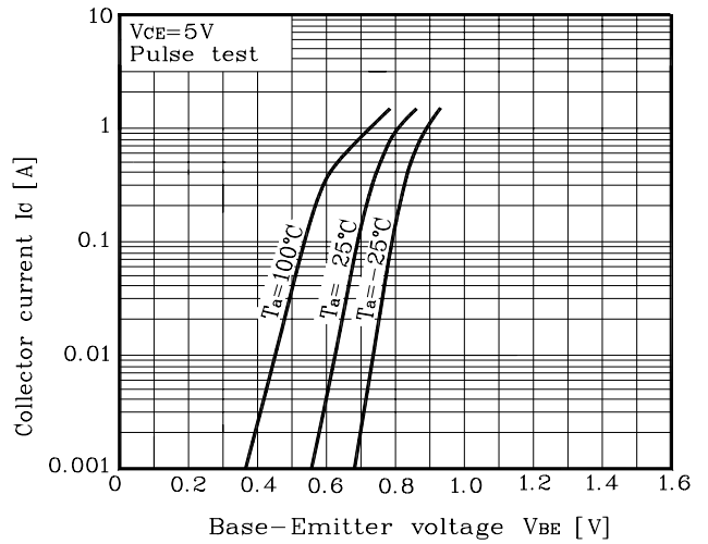
Fig. 2 I_C - V_{BE}
