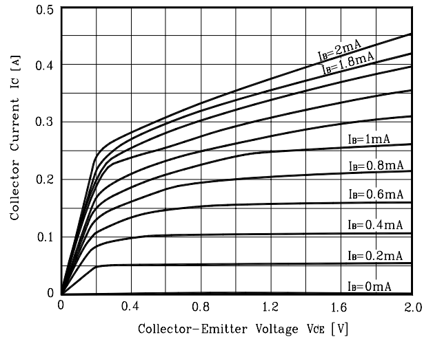
Fig. 4 I_C - V_{CE}
