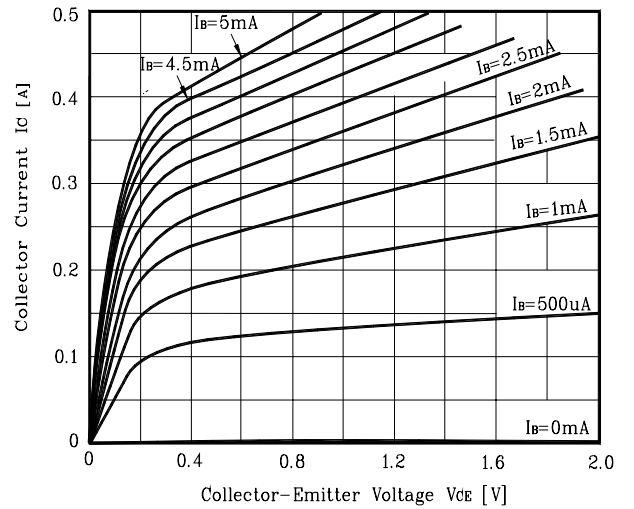
Fig. 4 I_C - V_{CE}
