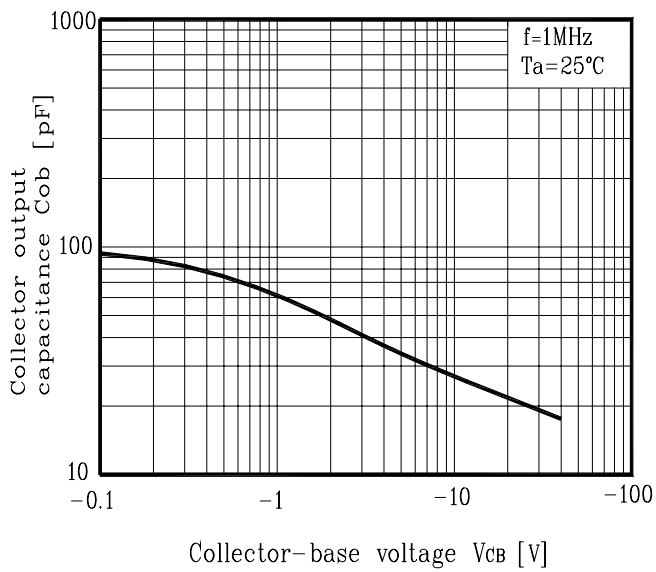
Fig. 7 C_{ob} - V_{CB}
