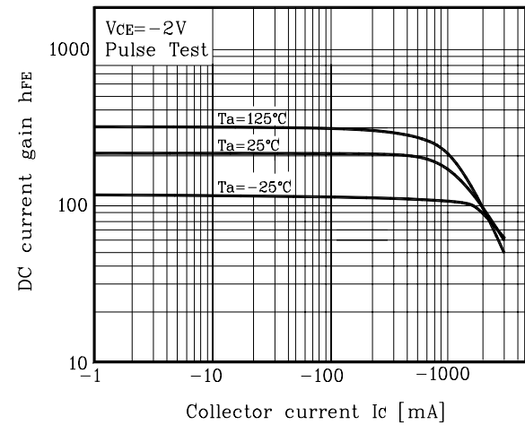
Fig. 4 h_{FE} - I_C
