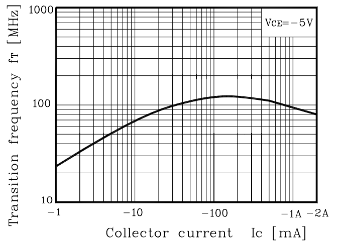
Fig. 4 f_T - I_C
