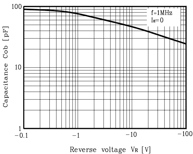
Fig. 5 C_{ob} - V_R
