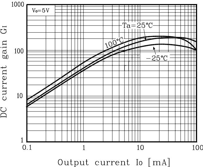
Fig. 3 G_I - I_O
