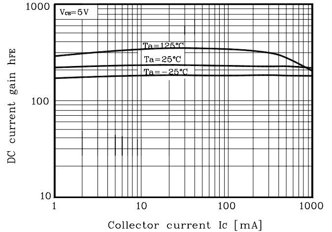
Fig. 8 h_{FE} - I_C
