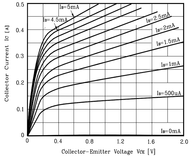
Fig. 4 I_C - V_{CE}
