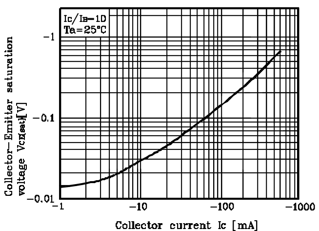
Fig. 5 V_{CE(sat)} - I_C
