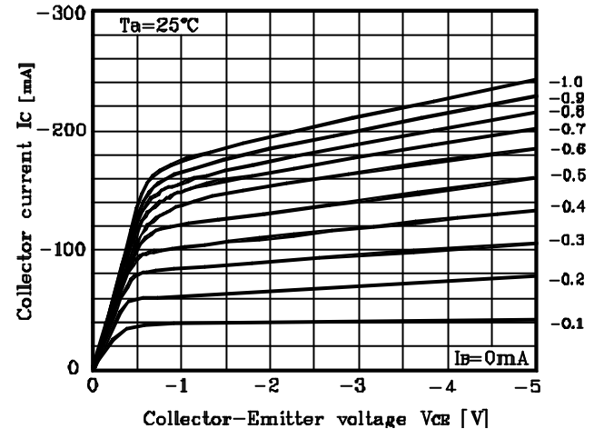
Fig. 4 I_C - V_{CE}
