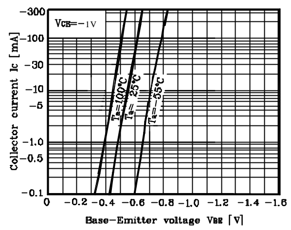
Fig. 2 I_C - V_{BE}
