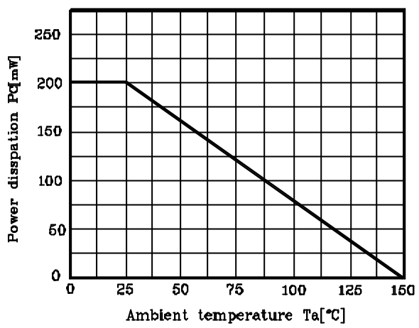
Fig. 1 P_C - T_a
