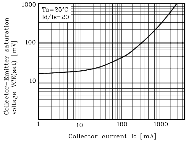
Fig. 4 V_{CE(sat)} - I_C
