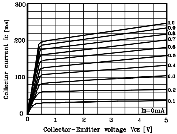
Fig. 4 I_C - V_{CE}
