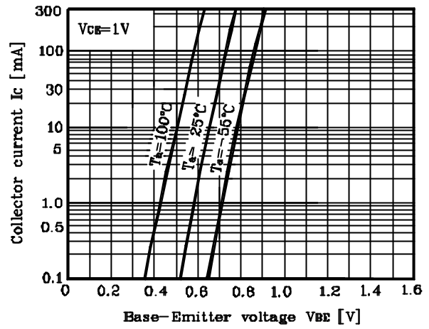
Fig. 2 I_C - V_{BE}
