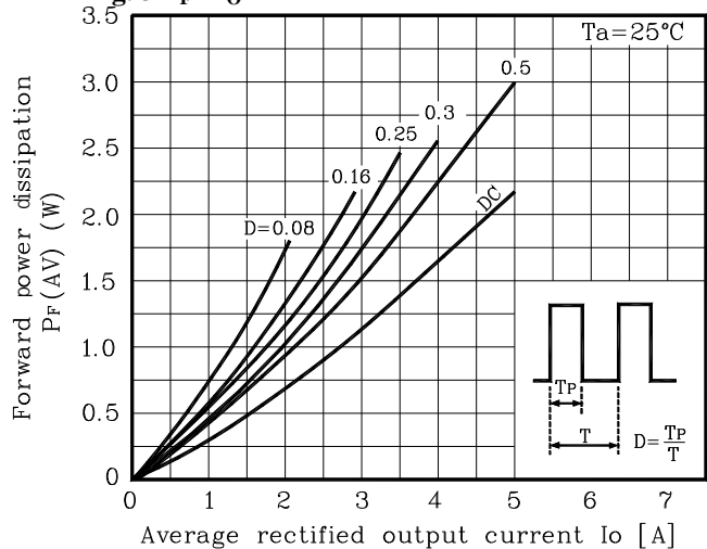
Fig. 3 P_F - I_O
