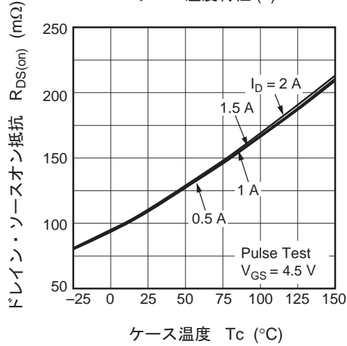
ドレイン・ソースオン抵抗対 ケース温度特性 (1)
