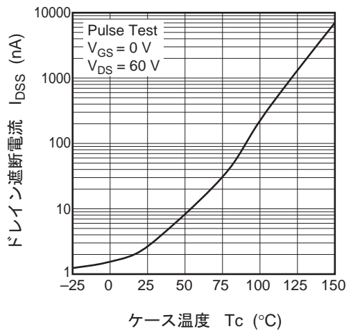
ドレイン遮断電流対ケース温度特性
