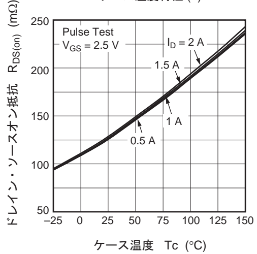
ドレイン・ソースオン抵抗対 ケース温度特性 (2)
