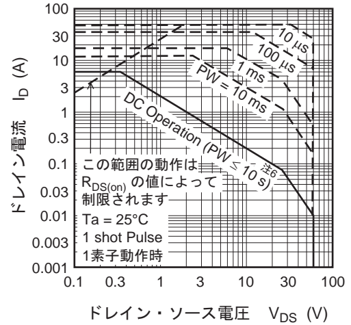
注6 ガラスエポキシ基板 (FR4 40 × 40 × 1.6 mm) 使用時の許容値
