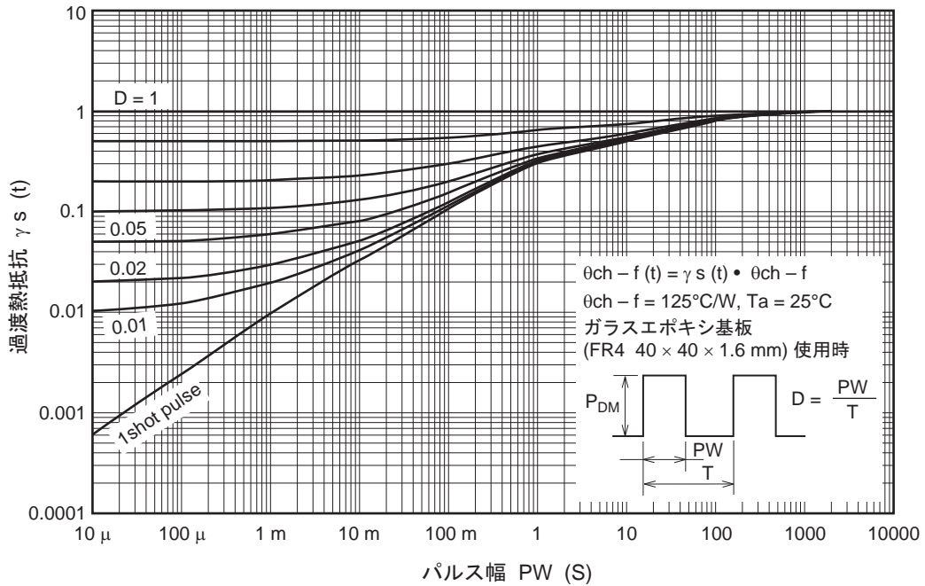
動作時の規格化過渡熱抵抗特性
