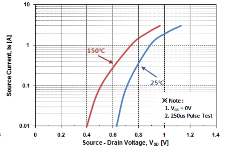
Fig. 4 I_S - V_{SD}
