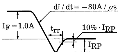
t_{rr} 波形
