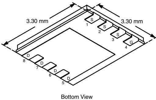
PowerPAK 1212-8
