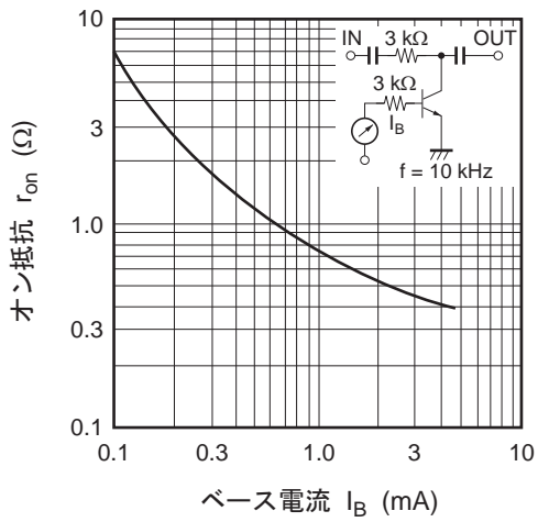
オン抵抗対ベース電流特性
