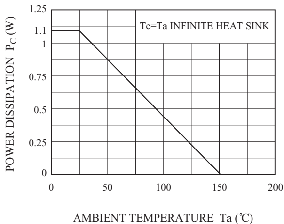
P_C - T_a
