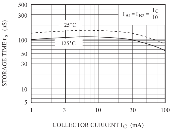
t_s - I_C
