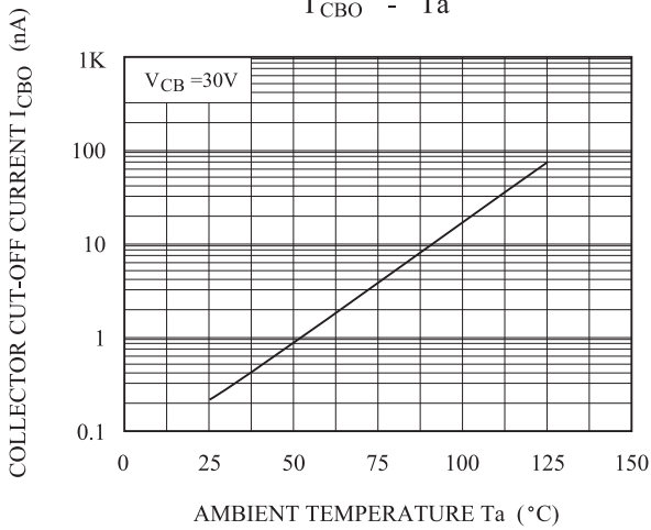
I_{CBO} - T_a
