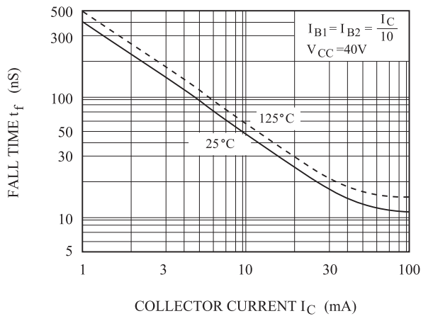
t_f - I_C
