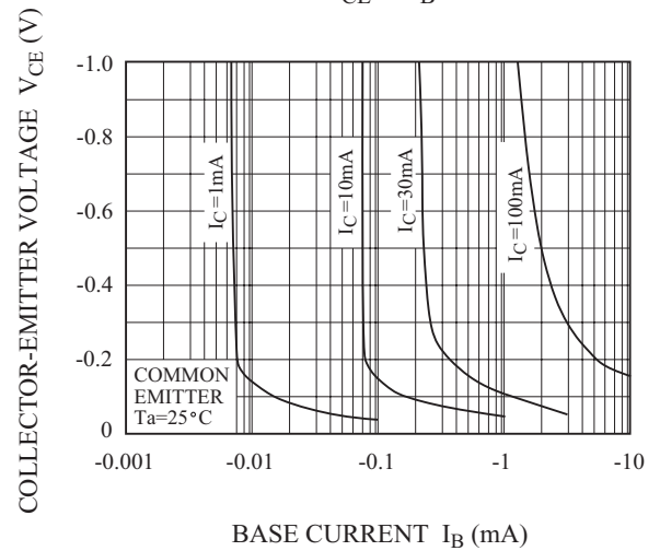
V_{CE} - I_B
