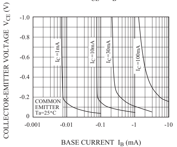
V_{CE} - I_B
