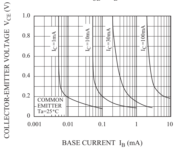
V_{CE} - I_B
