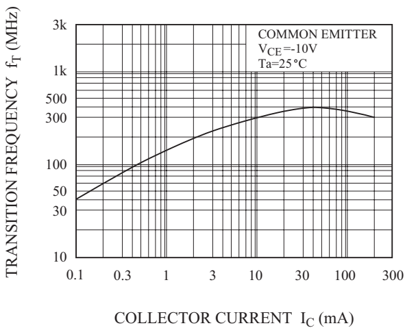
f_T - I_C
