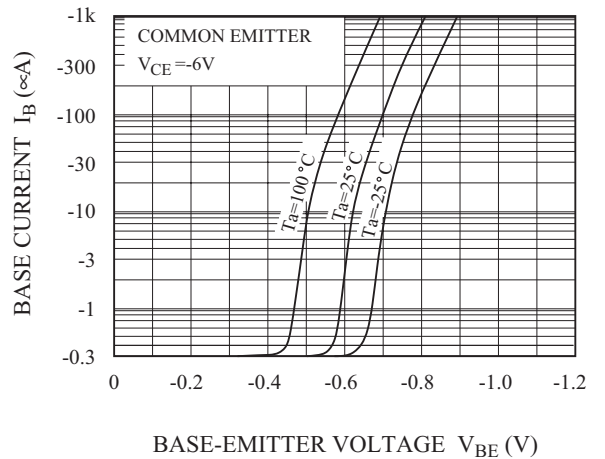
I_B - V_{BE}
