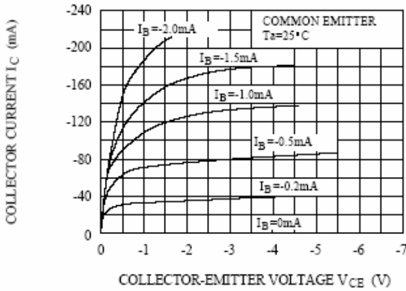
I_C - V_{CE}
